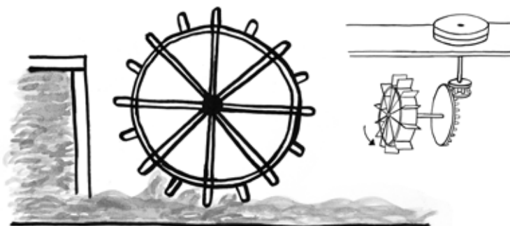
Jednoduchý vodní mlýn na spodní vodu. Převodové soukolí spojuje vodní kolo s horizontálními mlýnskými kameny.
